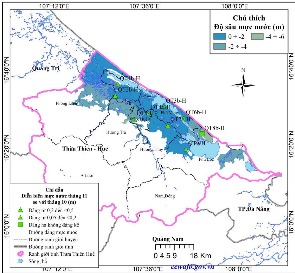
Hình 2. Sơ đồ diễn biến mực nước tháng 11 tăng qđ
